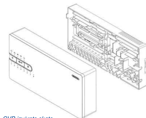
CVB izvērsts skats
